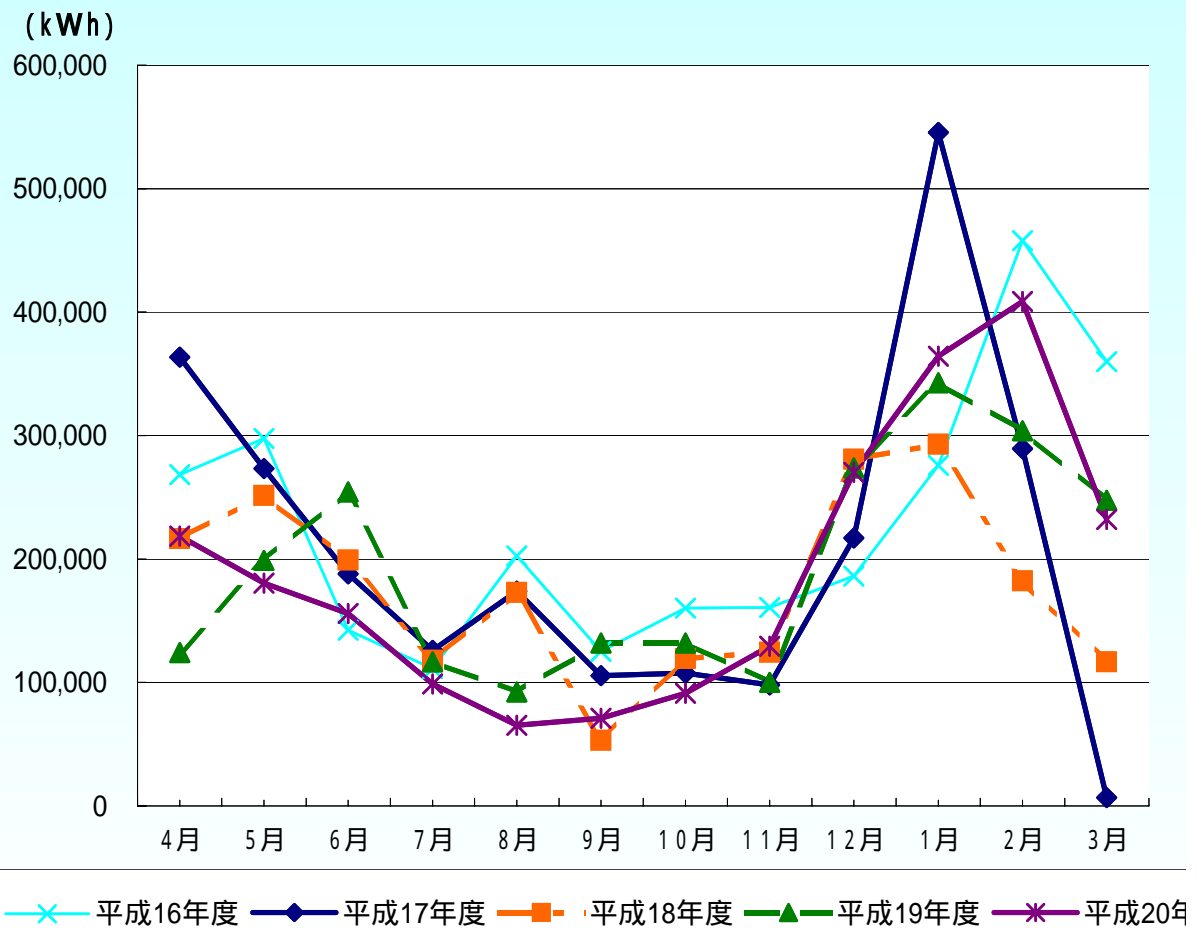
内灘町風力発電所月別売電量(表8 - 4参照)
