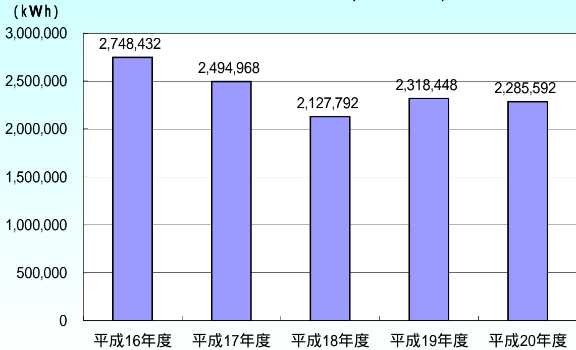
内灘町風力発電所売電量の推移(表8 - 4参照)
