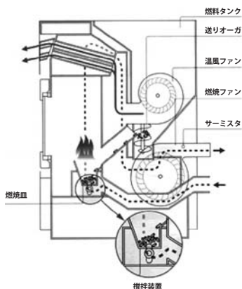
ペレットストーブのしくみ
