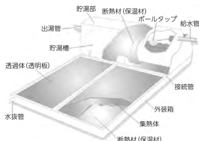
太陽熱温水器（自然循環型）
